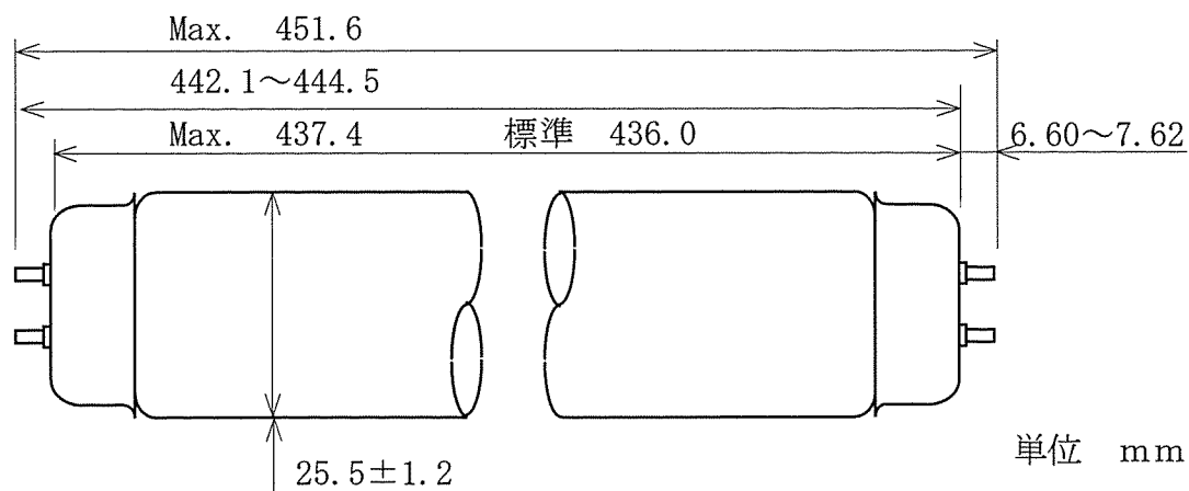
3波長形蛍光ランプ あかりん棒 〈ハイルミック〉
